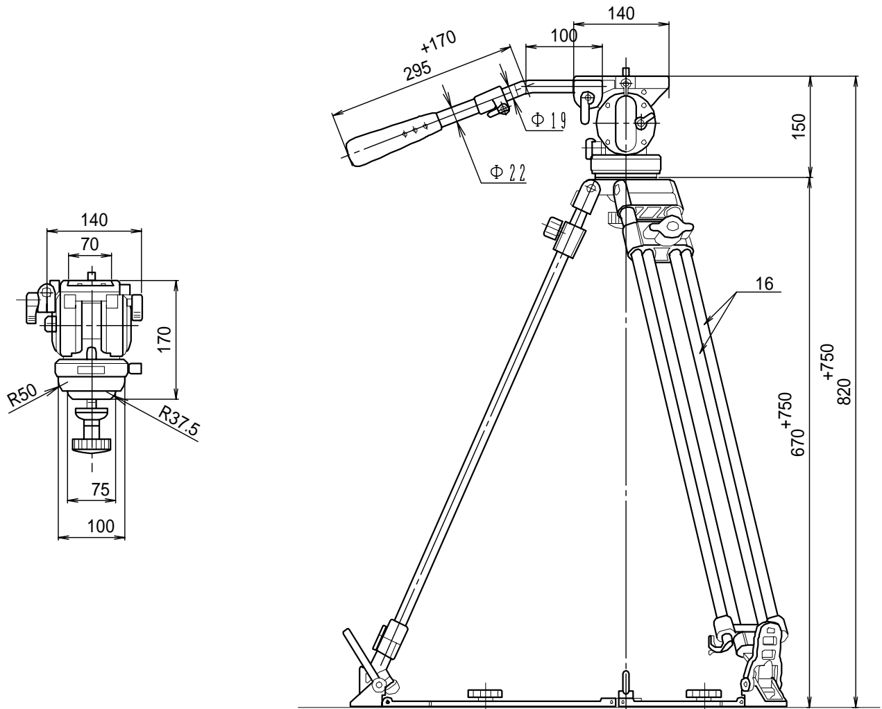
外觀寸法図[単位:mm]
