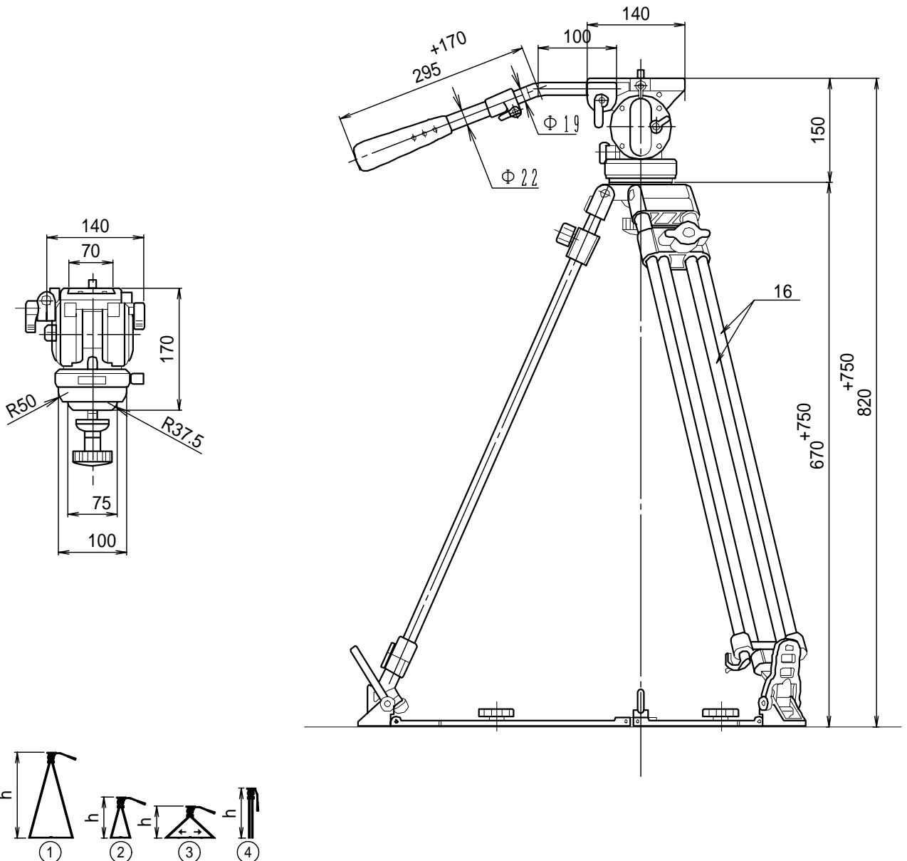
外觀寸法図[単位:mm]
