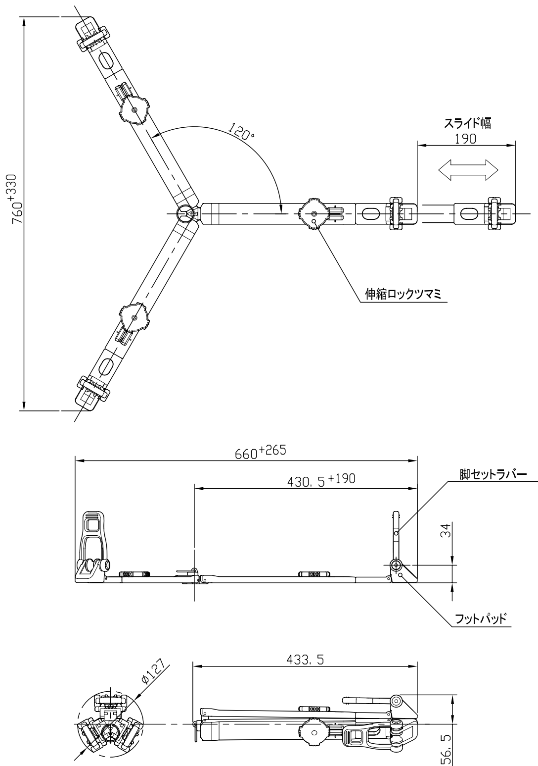
■外観寸法図[単位:mm]
