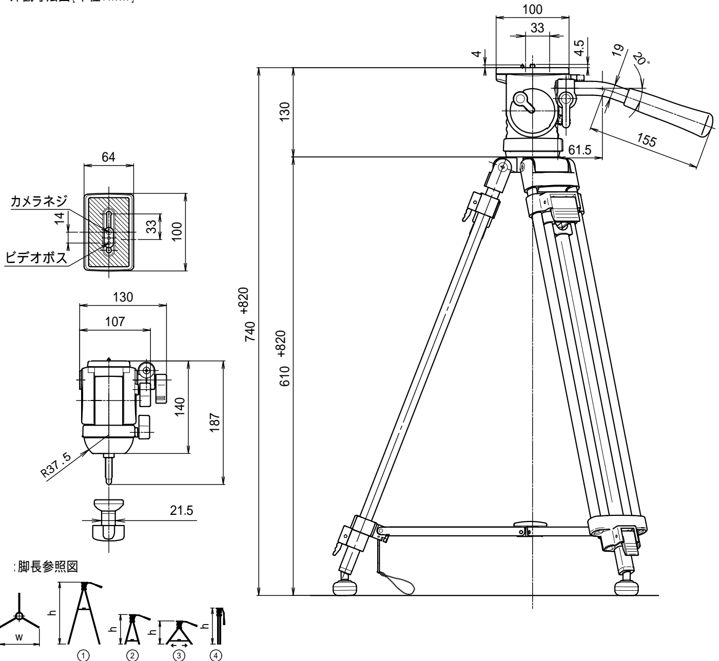
外観寸法図 [単位: mm]
