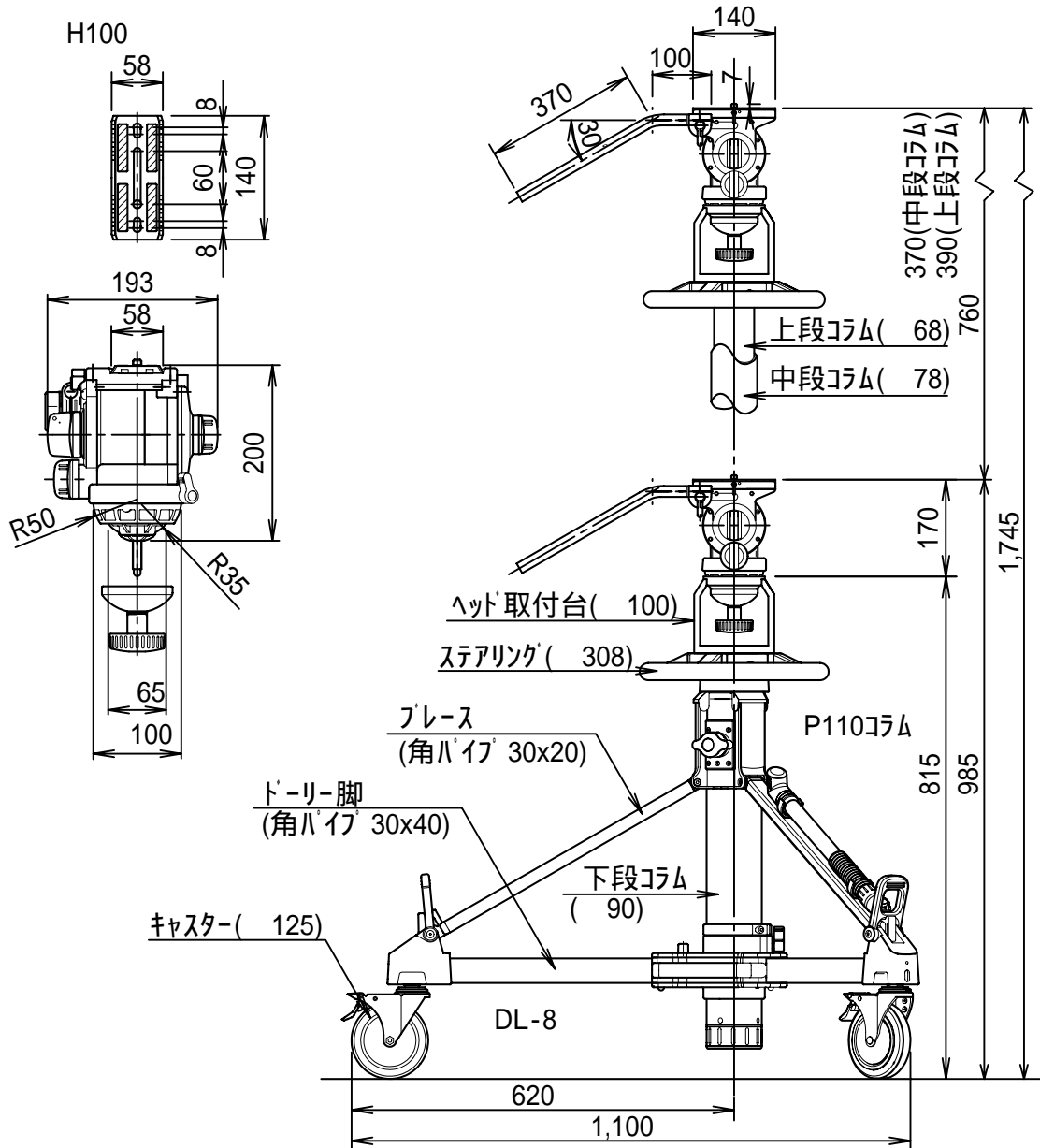
外観寸法図[単位:mm]
