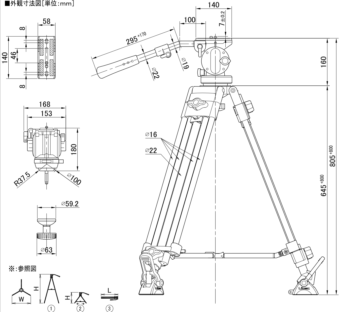
■外観寸法図[単位:mm]
