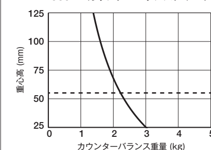
650EX カウンターバランスチャート
