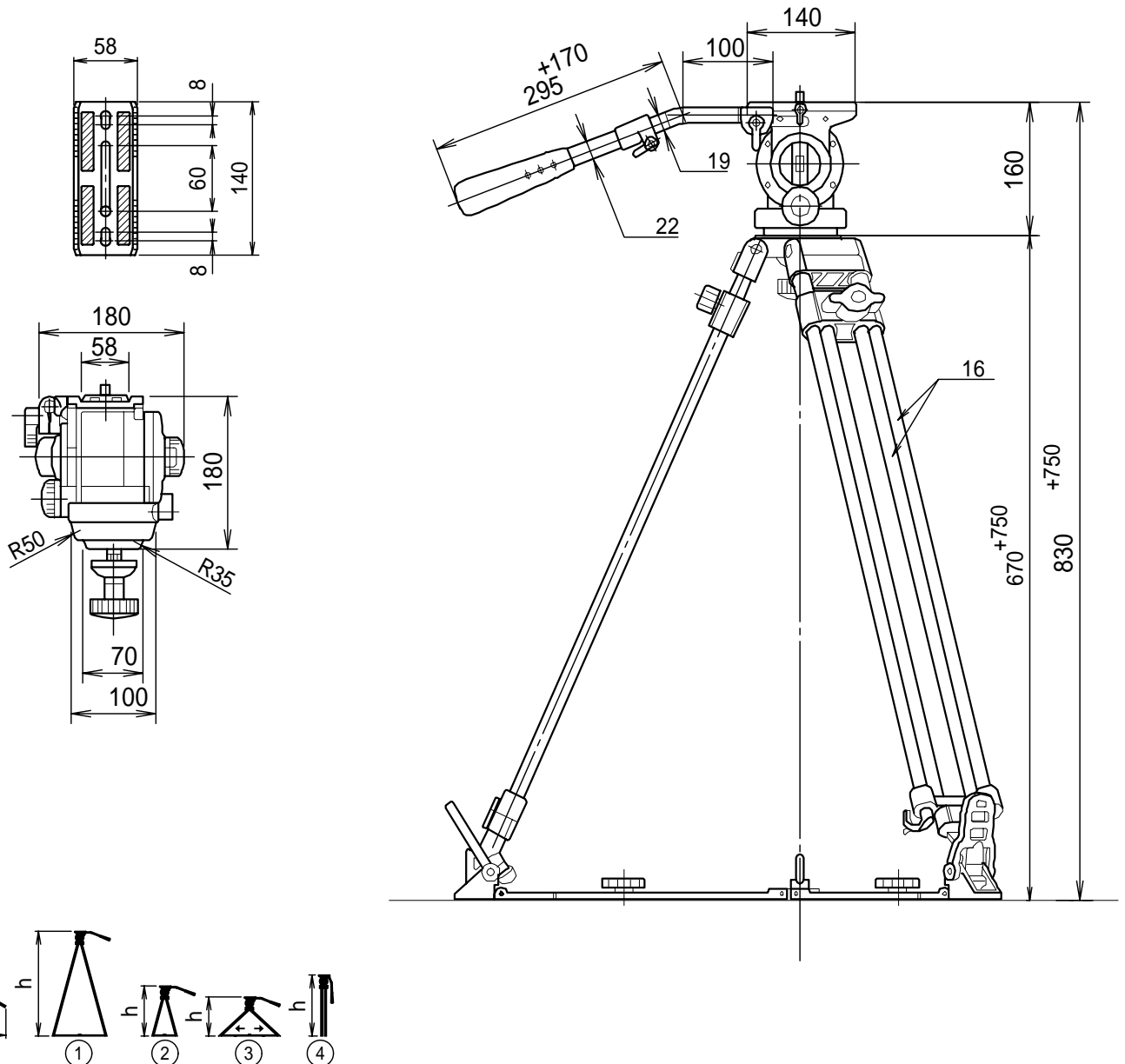
外觀寸法図[単位:mm]
