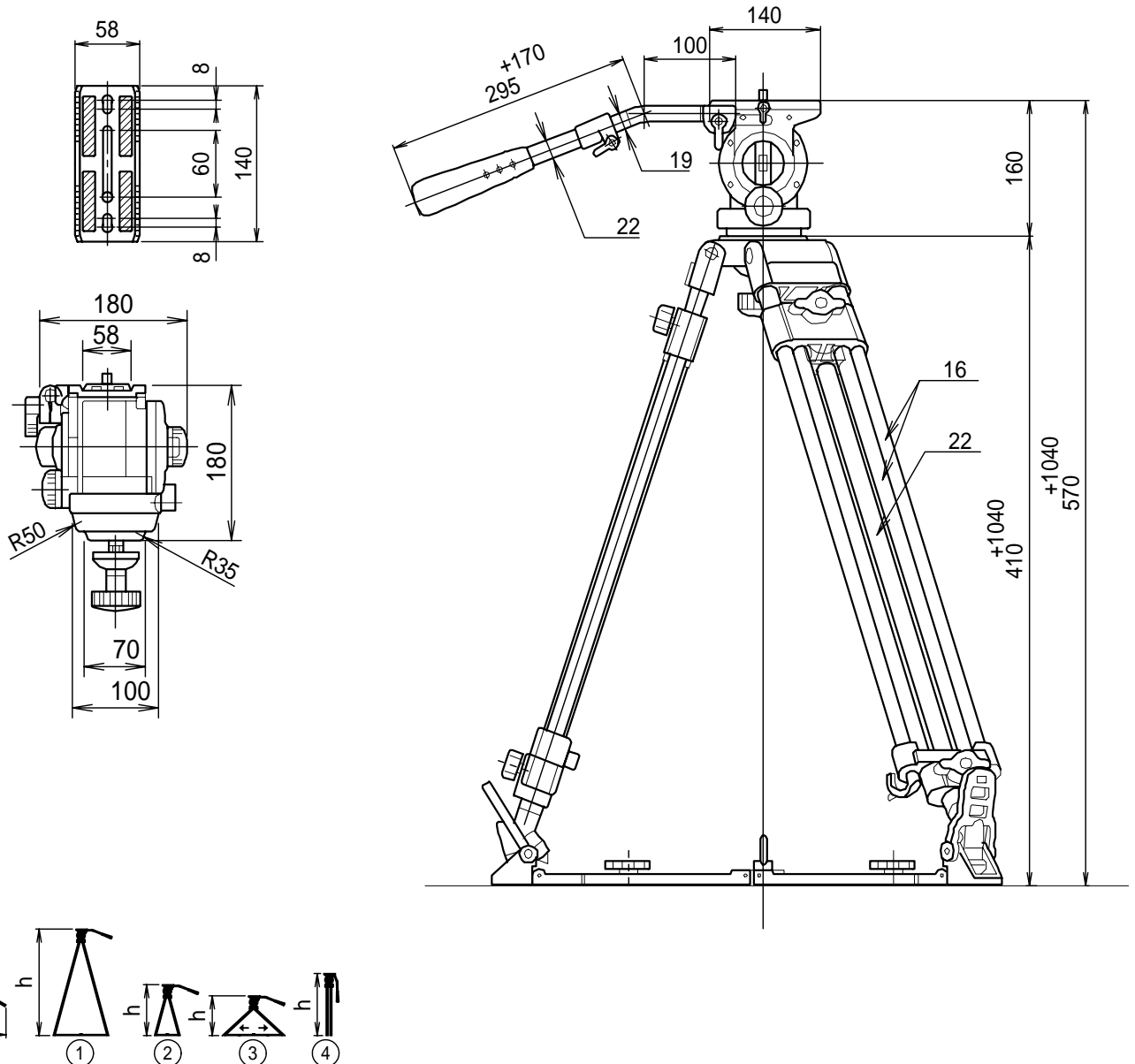
外觀寸法図[単位:mm]
